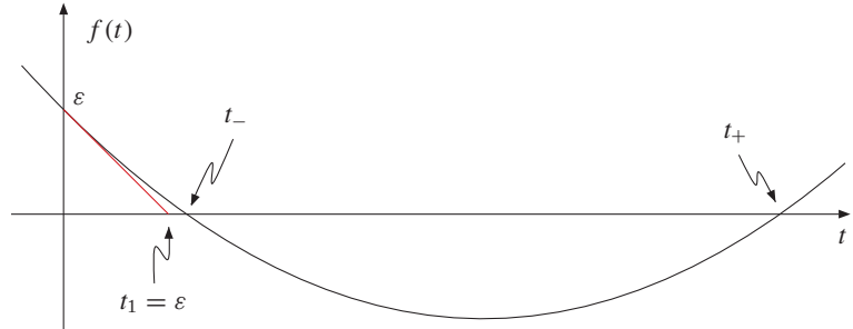
Figur 3.3.1 Første iterasjon av Newtons metode for funksjonen f(t)
